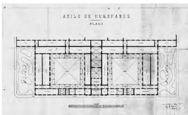
Plano Planta General
